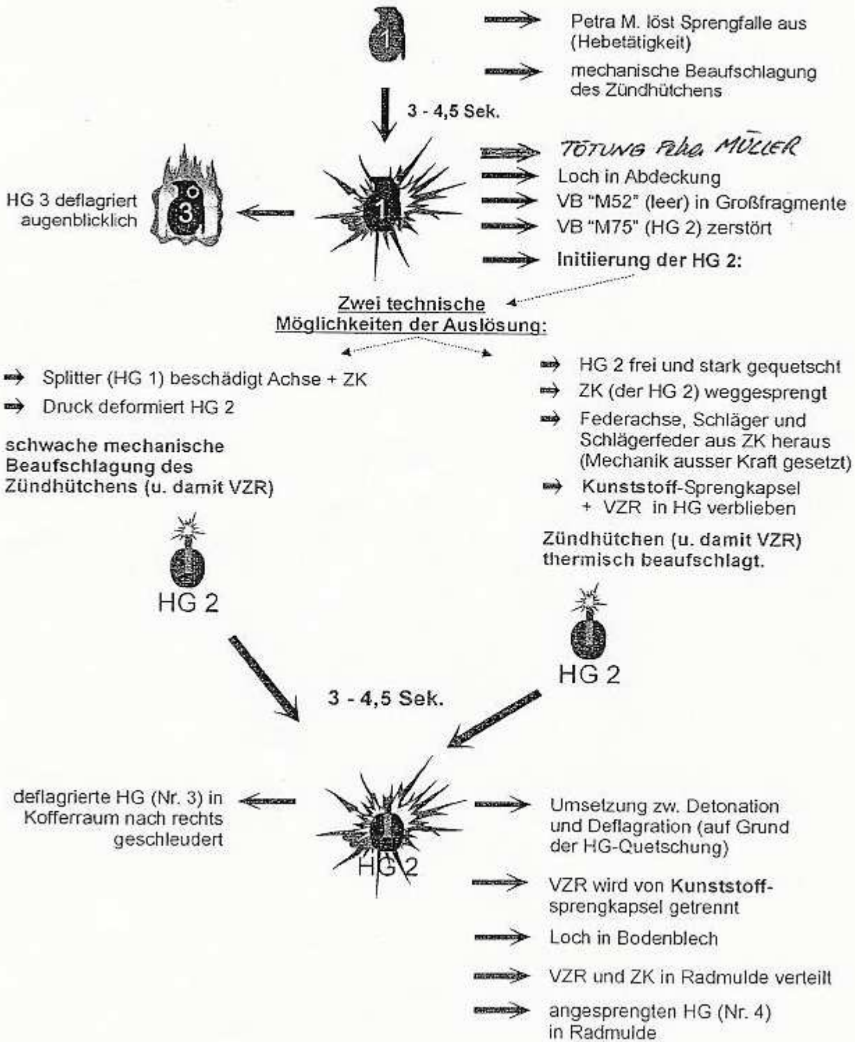
Abbildung 65: Ablaufdarstellung der Detonationen
